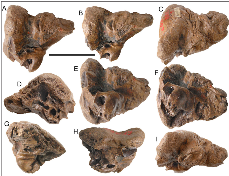
Fig. 12 - Specimen M. 652, right periotic. A) ventrolateral view; B) lateral view; C) dorsal view; D) medial view; E) ventral view; F) ventromedial view; G) anterior view; H) posterior view; I) dorso-lateral view. Scale bar equals 5 cm.
