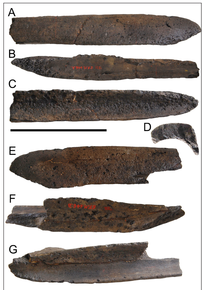
Fig. 23 - Mysticeti gen. et sp. indet. Specimen M. 646a, anterior end of right maxilla or premaxilla: A) dorsal; B) lateral; C) ventral views; D) natural cross-section at posterior end. Specimen M. 646b, anterior end of left maxilla or premaxilla: E) dorsal; F) Lateral; G) ventral views. Scale bar equals 10 cm.
