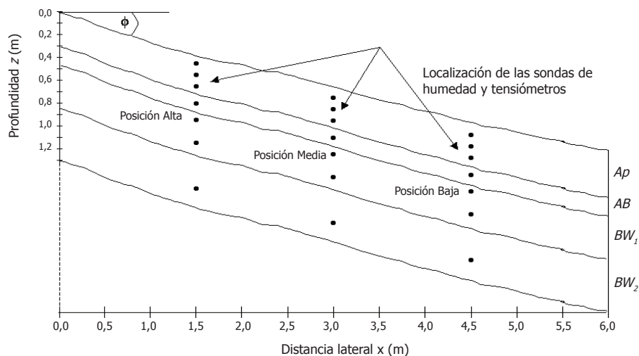
Figura 1. Ubicación de las baterías de sensores de humedad y de los tensiómetros en los monolitos aislados para estudiar la dinámica de los Andisoles bajo condiciones de ladera.
