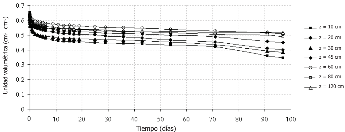
Figura 2. Evolución del contenido de humedad en los suelos unidad Chinchiná y unidad Montenegro, a lo largo del periodo de drenaje.
