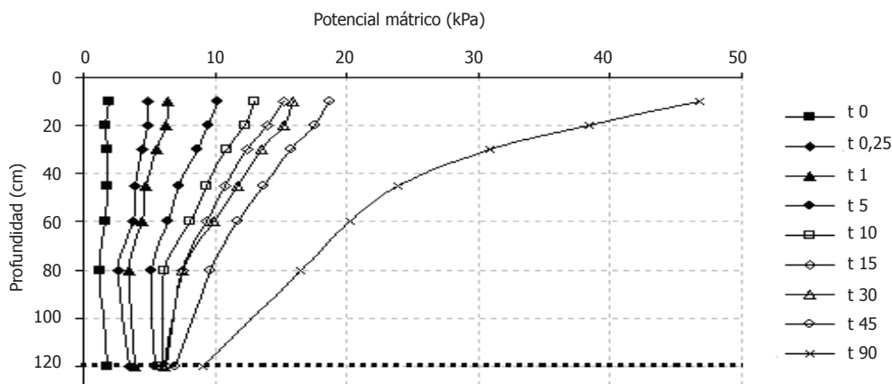
Figura 3. Comportamiento del potencial mátrico ( h ) en los suelos unidad Chinchiná y unidad Montenegro a diferentes profundidades y en diferentes tiempos de medición
