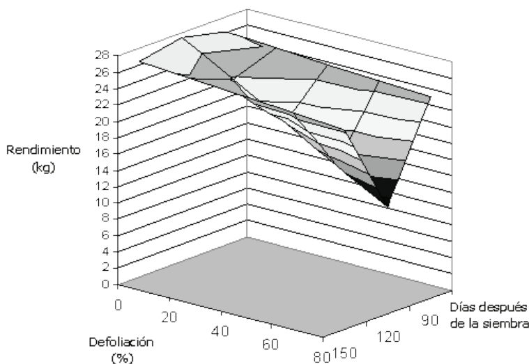
Figura 3. Superficie de respuesta para el rendimiento comercial en 25 plantas de papa cv. Parda Pastusa sometidas a diferentes niveles de defoliación.
