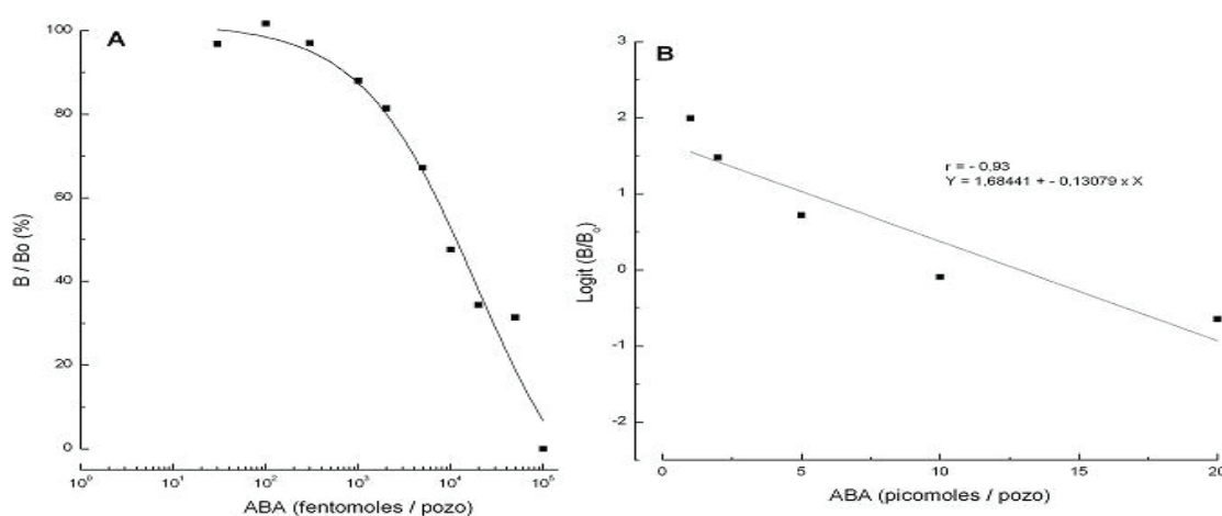
Figura 1. Curva patrón en función del porcentaje B/Bo y del logaritmo de la concentración de ABA en femtomoles/pozo (A) y datos transformados en una relación lineal usando la función logit de B/Bo (B).
