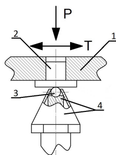
Рис. 2 – Контактна схема:
