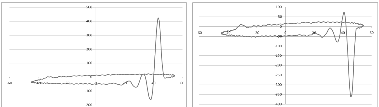
Рис. 4 – Петлі гістерезису в уординатах: переміщення верхнього контрзразка – тангенціального зусилля
