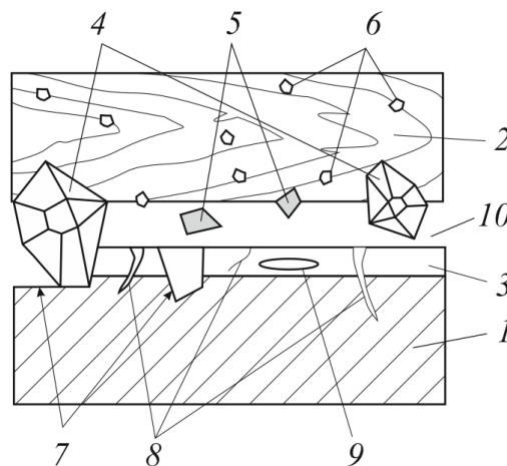
Рис. 1 – Схема фрикційної взаємодії у парі тертя «пресована тирса – сталь»:
