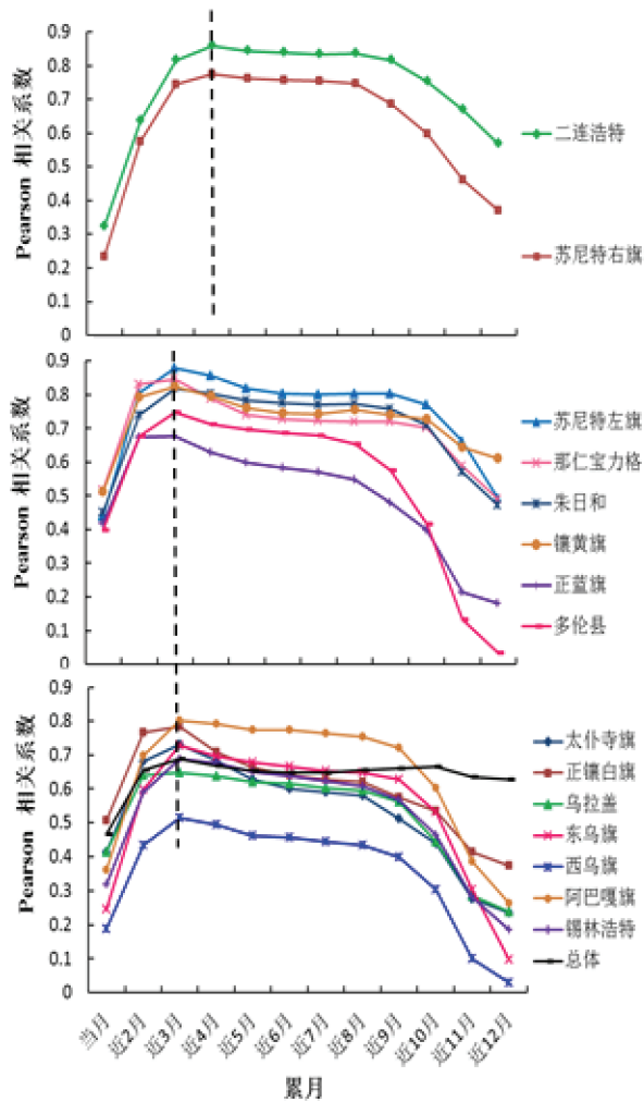
图 4. 生长季植被指数与累月降水量的相关系数
