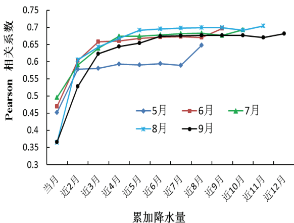
图 2. 各月 NDVI 与累月降水量的相关系数
