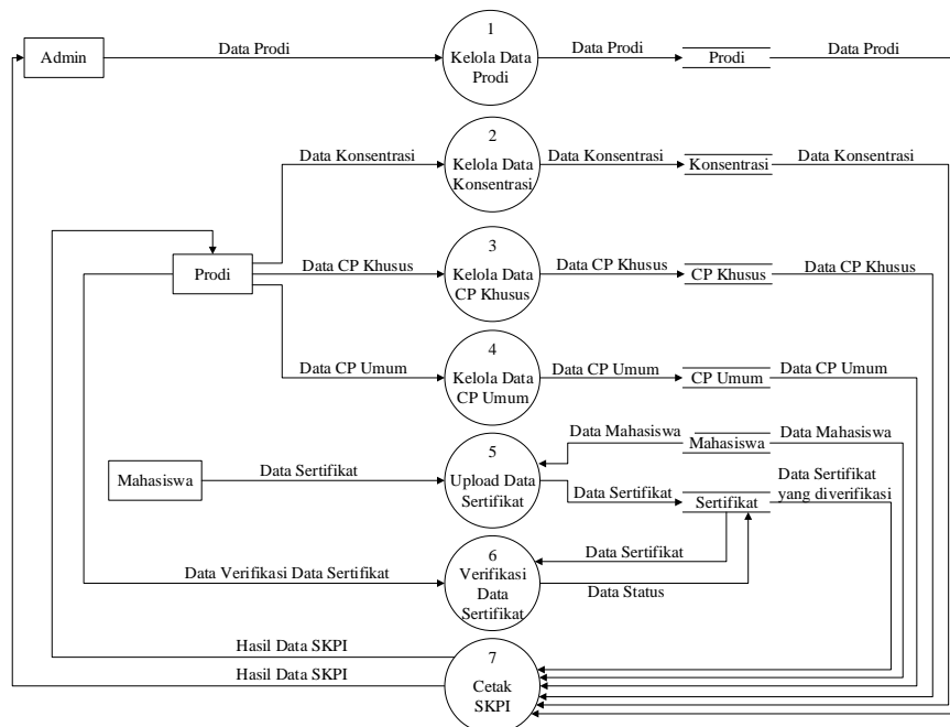
Gambar 3. DFD Level 0 Sistem E-SKPI Fakultas Teknik Universitas Islam Riau
