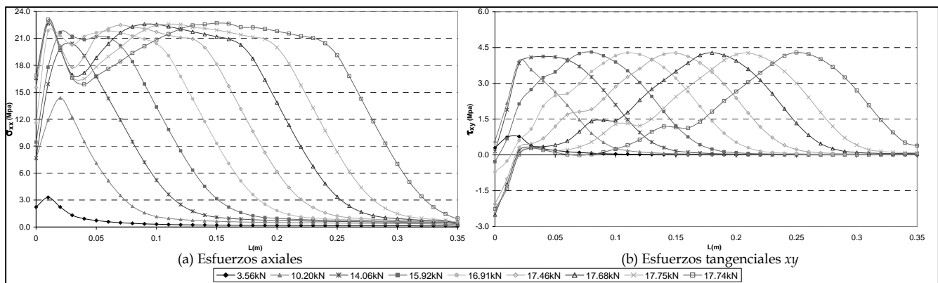
Figura 9. Distribución de los esfuerzos en el epoxy
