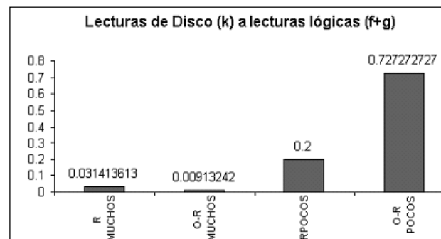
Figura 4. Tasa de lecturas de disco a lecturas lógicas para GROUP BY sencillo
