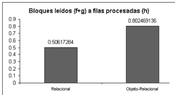
Figura 10. Tasa de bloques leídos a filas procesadas para las consultas con auto-reunión.
