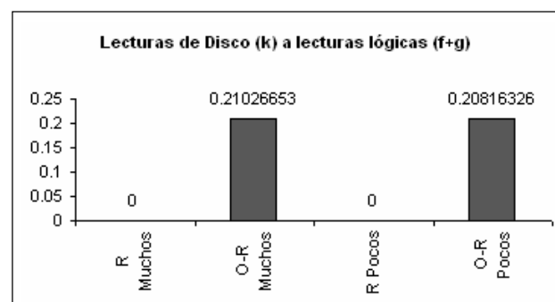
Figura 14. Tasa de lecturas de disco a lecturas lógicas para la reunión sencilla
