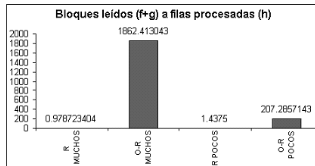
Figura 7. Tasa de bloques leídos a filas procesadas para las subconsultas cuando se utiliza la cláusula EXISTS
