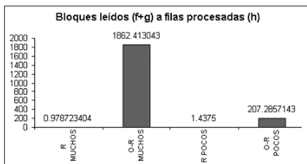
Figura 8. Tasa de bloques leídos a filas procesadas para las subconsultas cuando se utiliza la cláusula IN
