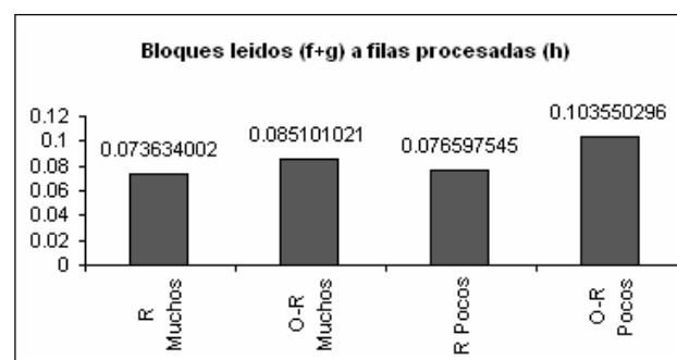
Figura 13. Tasa de bloques leídos a filas procesadas para la reunión sencilla
