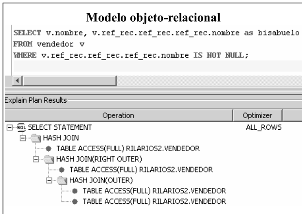
Figura 9. EXPLAIN PLAN para los modelos relacional y objeto-relacional para la consulta e auto-reunión
