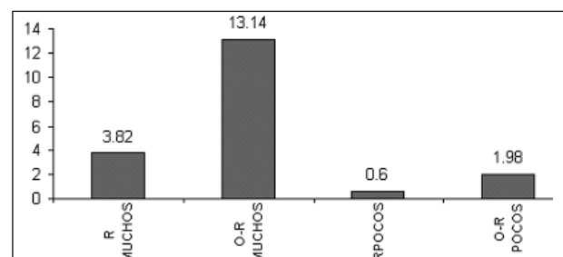
Figura 3. Tasa de bloques leídos a filas procesadas para GROUP BY sencillo
