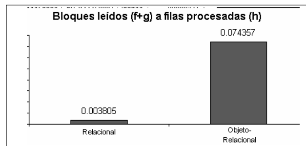
Figura 11. Tasa de bloques leídos a filas procesadas para las pruebas con el Modelo 2
