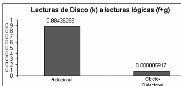
Figura 12. Tasa de lecturas de disco a lecturas lógicas para las pruebas con el Modelo 2
