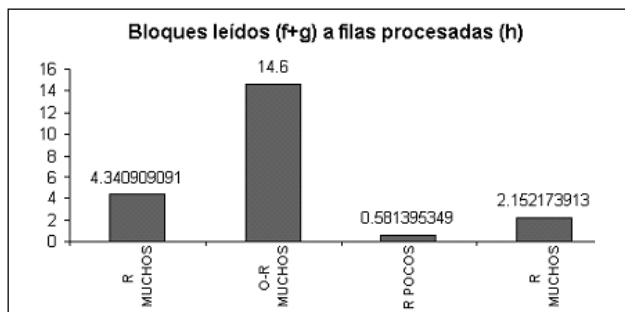
Figura 5. Tasa de bloques leídos a filas procesadas para GROUP BY con las cláusulas HAVING y ORDER BY
