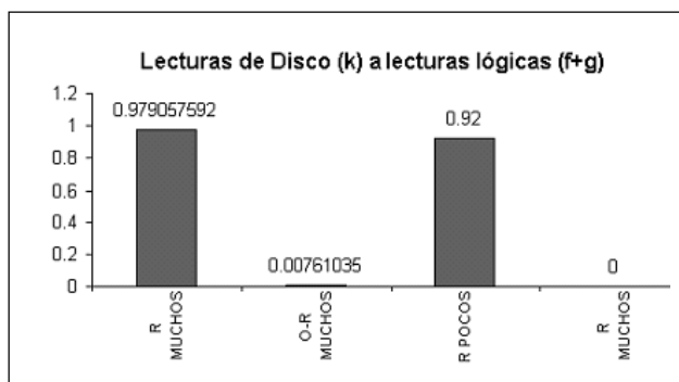
Figura 6. Tasa de lecturas de disco a lecturas lógicas para GROUP BY con las cláusulas HAVING y ORDER BY
