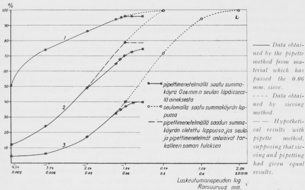
Piirros 1. Mekaanisen maa-analyysin summakäyriä. 1. Hiesusavi. 2. Hiesuinen hietä. 3. Hietamoreenin alle 2 mm:n aines.
